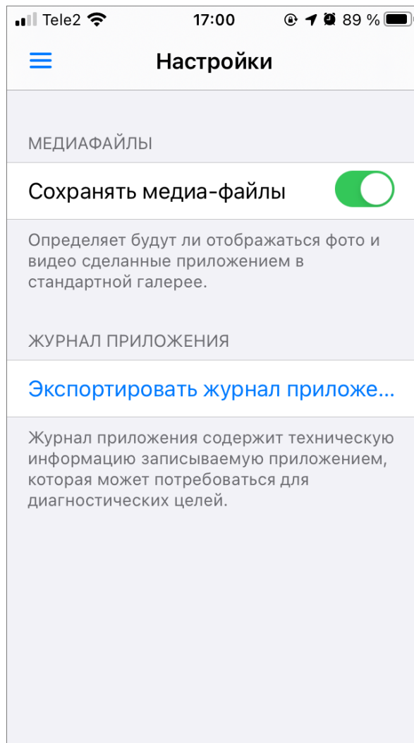
Рис. 17 Окно «Настройки»
