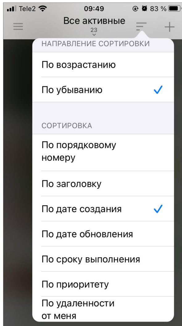
Рис. 8 Окно сортировки
