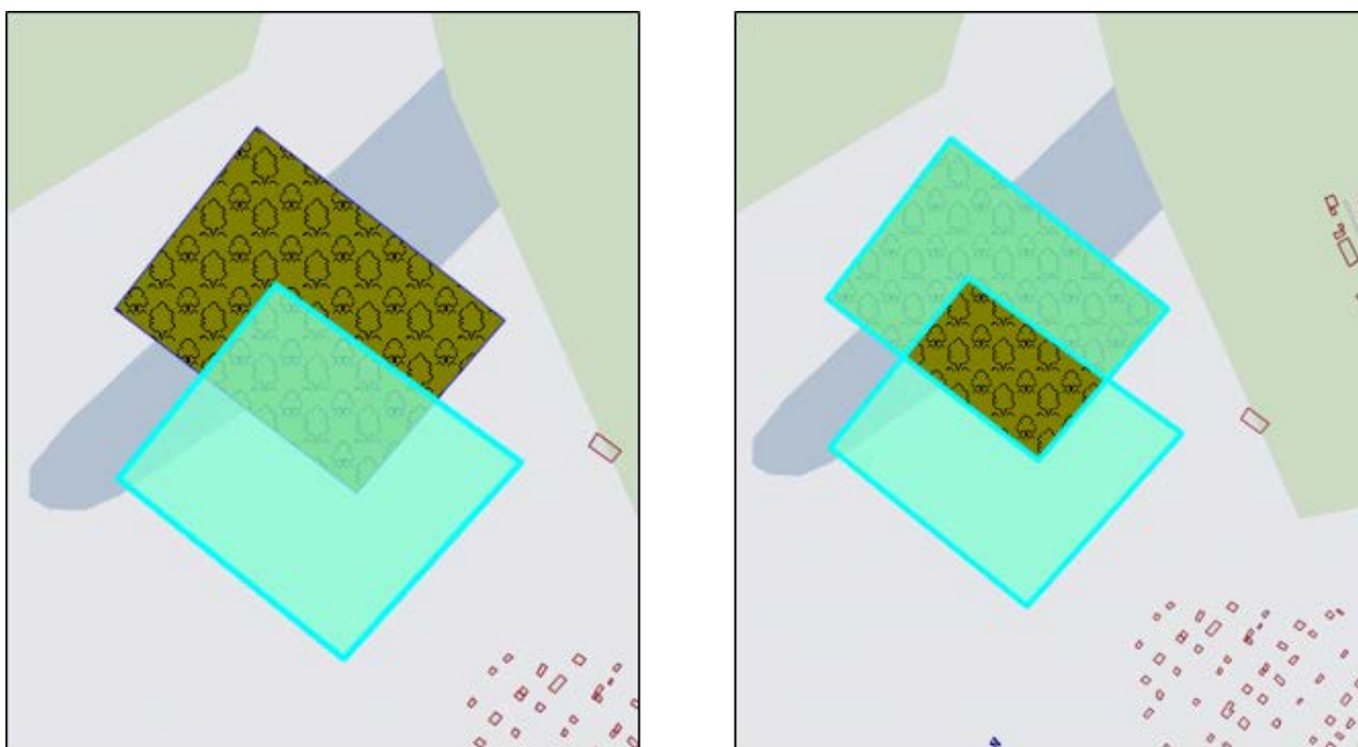
Рис. 138 Симметрическая разность двух полигонов
